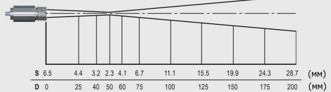
Оптика CT LT CF, D:S = 22:1 (вдали = 1.5 :1)
