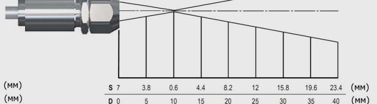
Оптика CT LT CF, D:S = 22:1 (вдали = 1.5 :1)
