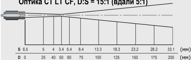
Версия со встроенными линзами CF Оптика CT LT CF, D:S = 15:1 (вдали 5:1)
