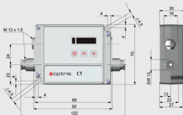
Размеры блока электроники
